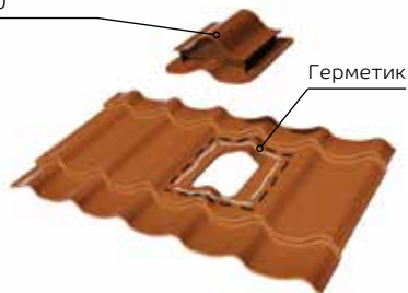
Вентилятор KTV Ø110
