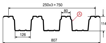
Профилированный лист Н-114x750-А
